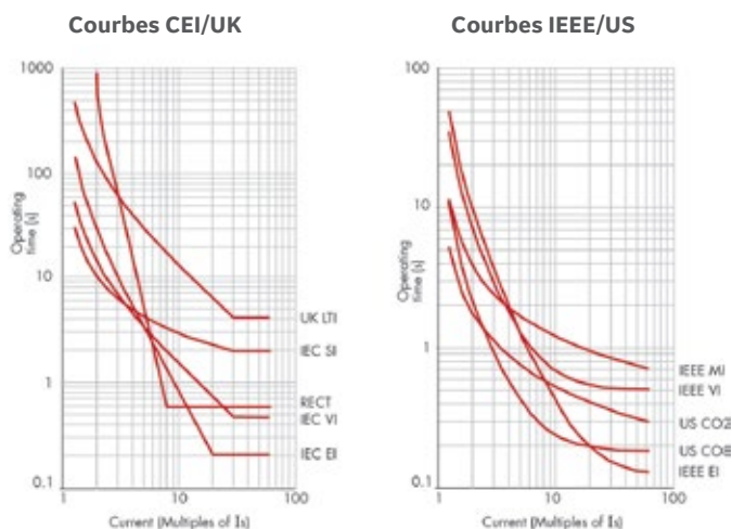
Profils de courbes à temps inverse CEI et ANSI/IEEE
